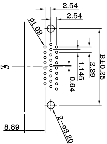
P.C.B LAYOUT
